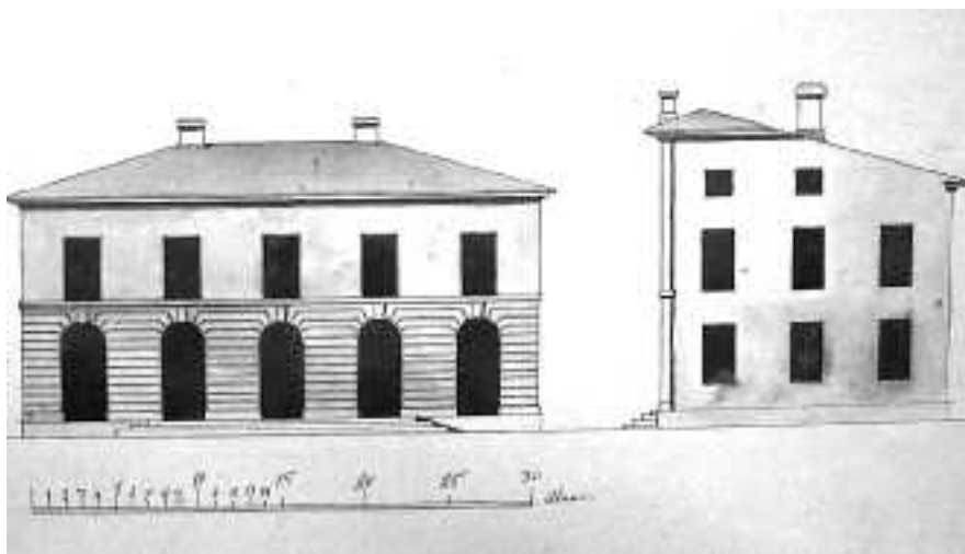
Apotekshuset, ritning till fasaden mot parken med de två övre våningarna på ett löst ark, möjligen av utförd av Gustav III.
