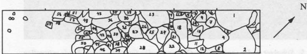
Fig. 8. Avvägningsplan, överförd från lodfotoplanen, över det framrensade övre stensiktet. Samtliga avvägningsbara stenar (58 st) har numrerats. Översättningstabell nedan med värden som anger höjden över Mälarens yta. Skala 1:50.
