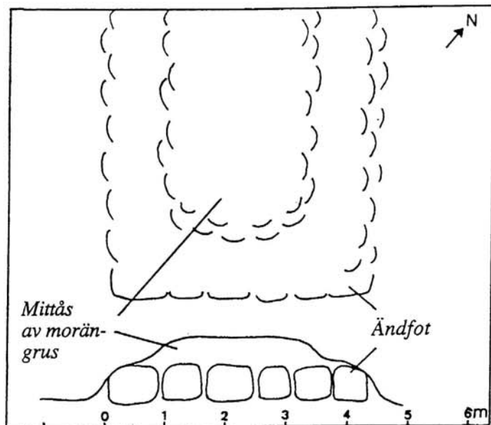
Fig.12. Principskiss av den längsgående mittåsens tvärsnitt - en tänkbar "palissadfyllning" - som kan skönjas i vallens Ö del och som till stora delar består av sintrat morängrus. Vallen avslutas med en ändfot (4,3 m bred) av 6 stenar som ligger på berget ca 2 m innanför stupet.
