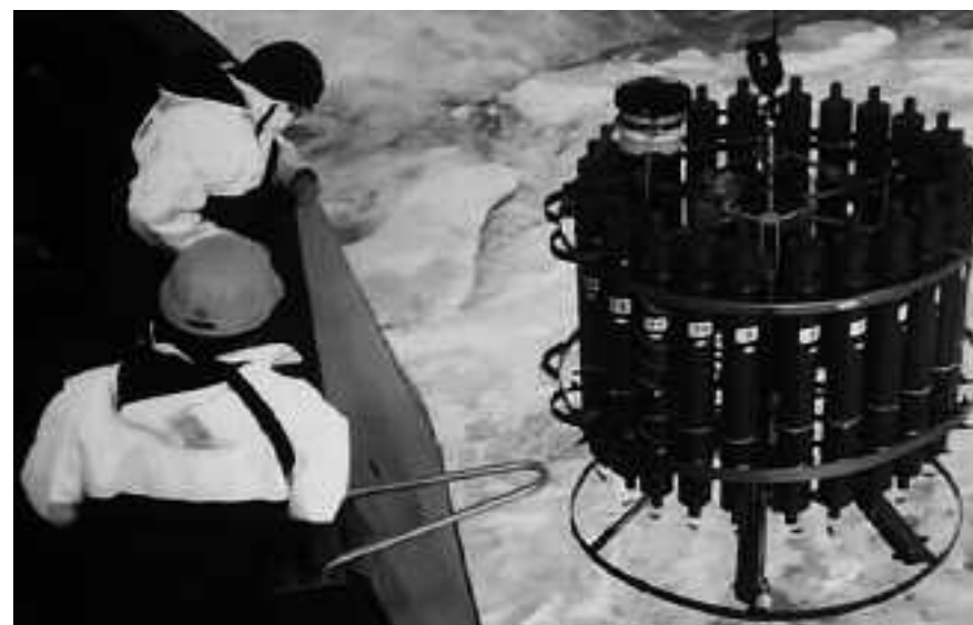
Bilder ur Jörgen Eks föredrag om klimatforskningen i Norra ishavet: Metangas lösgörs och bubblar upp från botten när vattentemperaturen stiger. Nedan: Utrustning för provtagning
